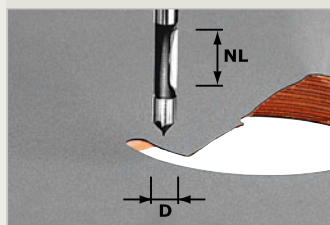
Fúrómaró
