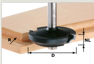
Lemunkáló maró golyócsapággal
