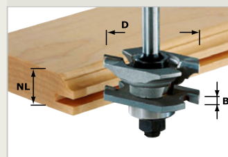
Profil-horony-maró
