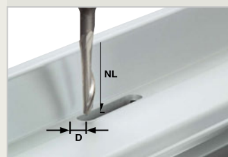
Alumínium maró
