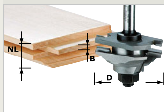
Profil-ereszték-maró
