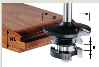
Ereszték ellenprofilmaró golyócsapággal
