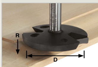
Lemunkáló maró golyócsapágý nélkül △ n max 22000
